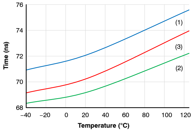
(1) t_{DIS} , V_{DD1} = 3.3\text{ V} (2) t_{DIS} , V_{DD1} = 5\text{ V} (3) t_{DIS} , V_{DD1} = 20\text{ V}
